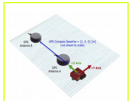
sposób działania kompasu GPS
