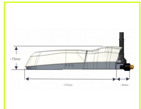
wymiary RELAY7 + SMART7
